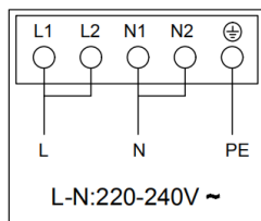
APV2303/AV3602
